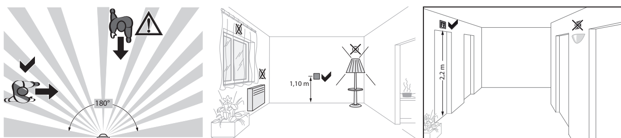
Bild 4: Montageort von Bewegungsmeldern
