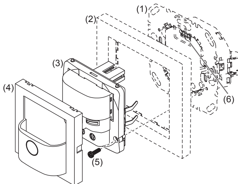
Bild 1: Geräteaufbau
