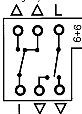
Koblingsskjema
