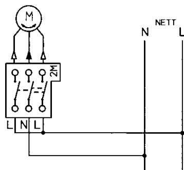
Målskisse
