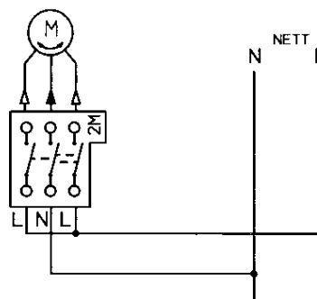
Koblingsskjema
