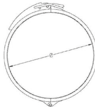
Diam 080-400 mm med ledat band.
