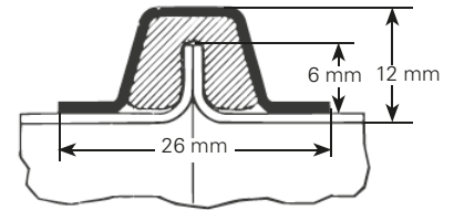
Skiss på anslutning av spännband för 0,6-1,25 mm galvplåtsdetaljer med spännbandskant (uppkragad).
