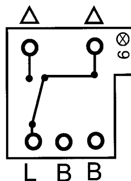
Koblingsskjema
