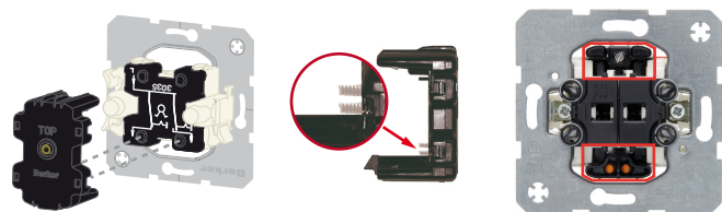
Bild 1: Das LED-Aggregat besitzt Kontaktfedern (s. Bild mitte), die das einfache Aufrasten von hinten gewährleisten
