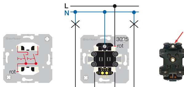
Bild 2: Serien-Kontrollschaltung (Aggregat leuchtet pro Serie bei „Ein“), N-Klemme (s. Bild rechts)
