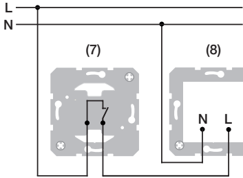
Bild 2: Anschlussbeispiel LED-Signallicht, weiße Beleuchtung
