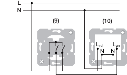
Bild 3: Anschlussbeispiel LED-Signallicht, rote/grüne Beleuchtung
