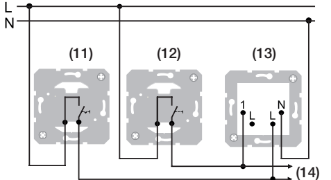
Bild 5: Anschlussbeispiel Farbumschaltung über Außenleiter, nicht geschleift
