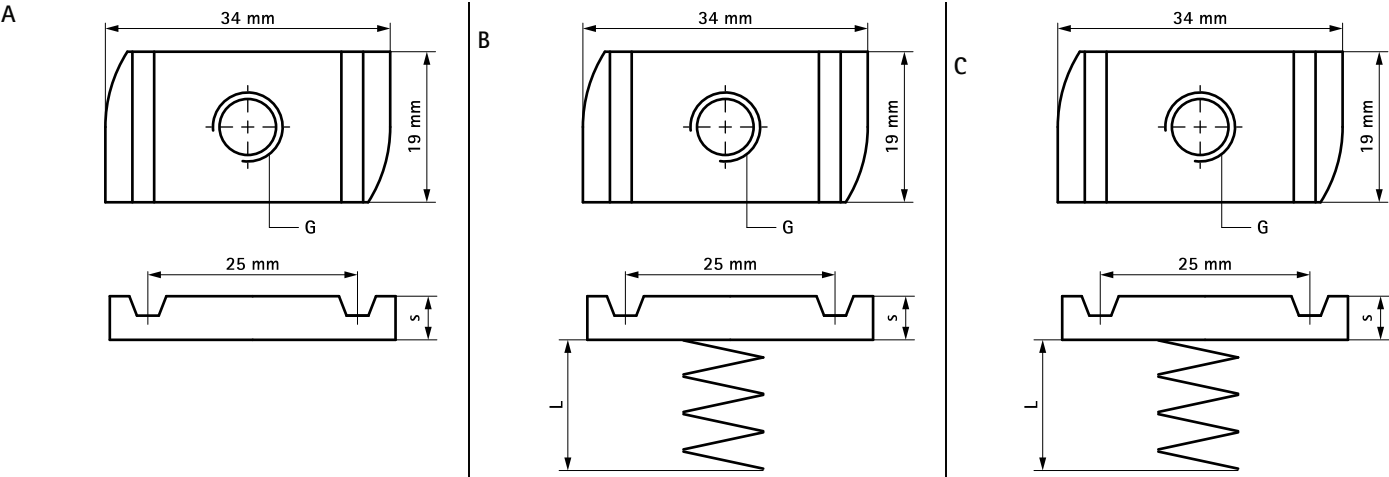
Alternative BIS Strut Slide Nut (BUP1000)
