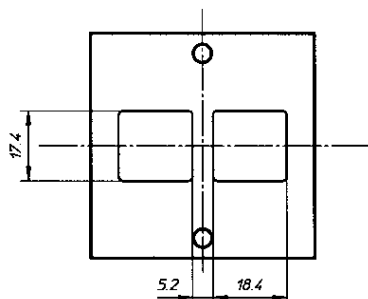
Målskisse
