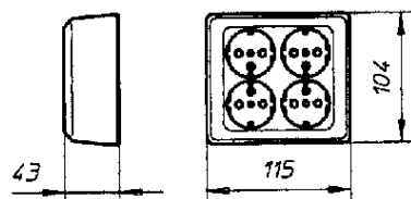
Målskisse
