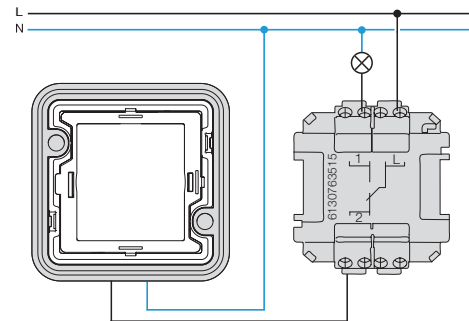
Bild 11: Beleuchtet bei AUS (Orientierungs-Beleuchtung), mit Wechselschalter, für z. B. Bedienstellen abseits vom Tageslicht wie in Kellern und Garagen
