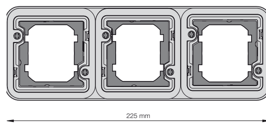
Bild 7: Rahmen 3fach für UP-Montage
