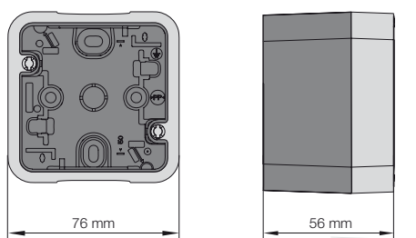
Bild 1: Gehäuse AP
