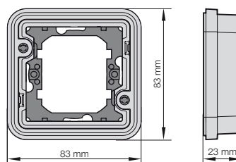
Bild 5: Rahmen 1fach für UP-Montage
