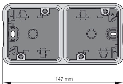
Bild 2: Gehäuse 2fach AP
