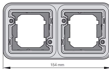
Bild 6: Rahmen 2fach für UP-Montage
