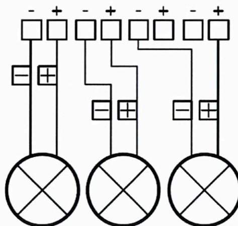
Kobling ved bruk av 3 downlights
