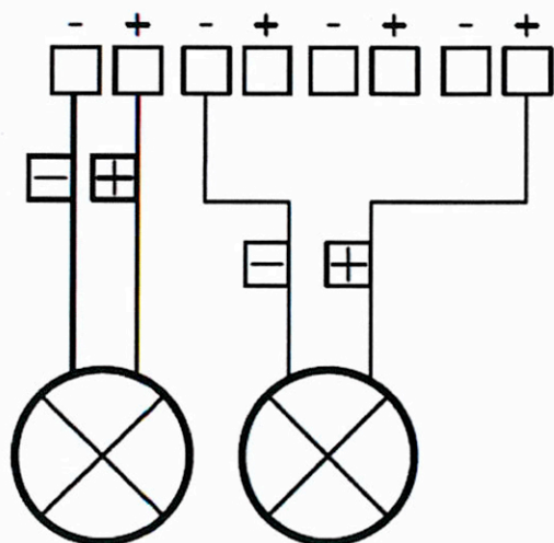
Kobling ved bruk av 2 downlights
