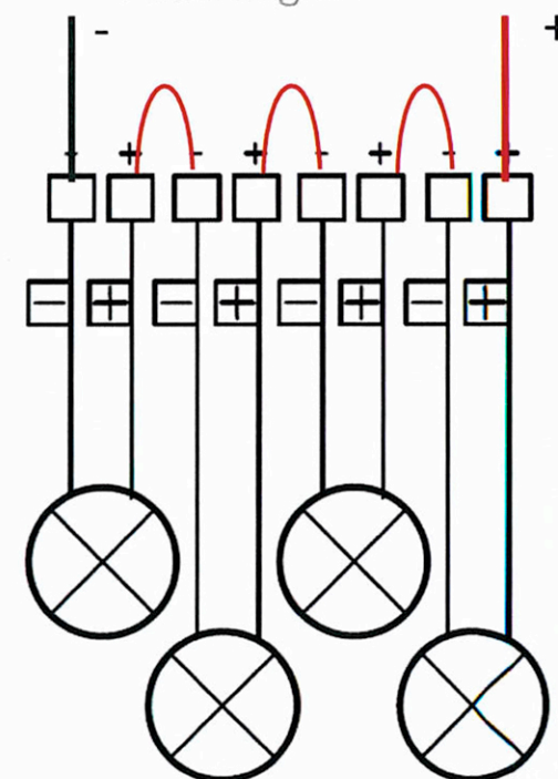
Kobling ved bruk av 4 downlights
